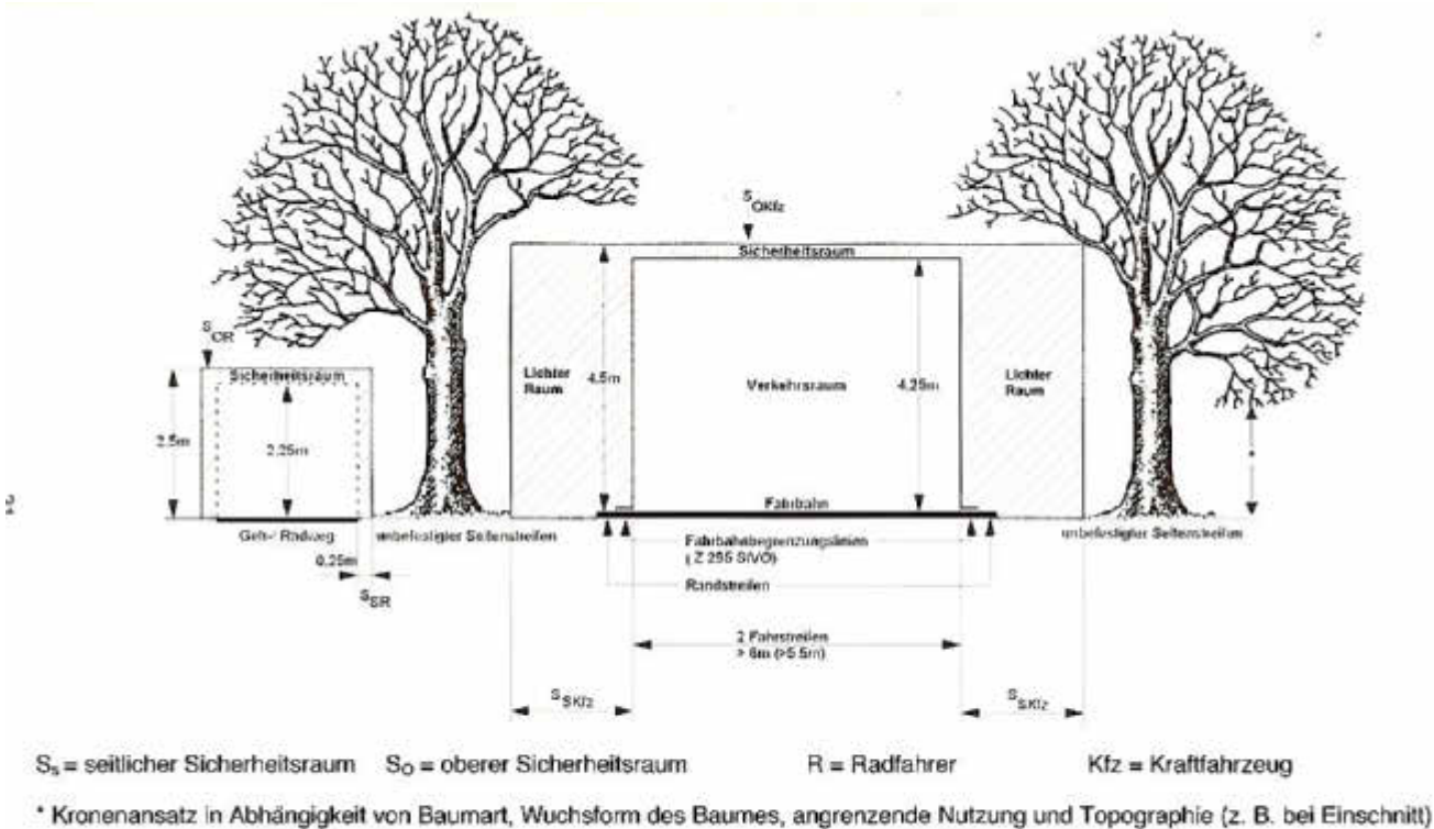
Abb. 2: Beispielhafte Darstellung des Lichten Raumes in Anlehnung an RAS-Q für anbaufreie Straßen
